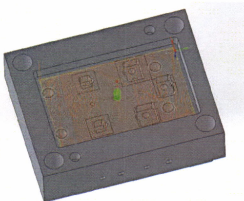
Werkstück mit Werkzeugwegen, erzeugt in i-Machining. Bild: DPS
