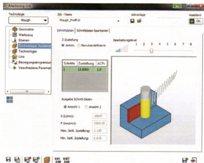
Eingabemaske für i-Machining. Bild: DPS
